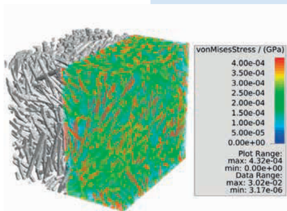
Von-Mises-Spannung in der Mikrostruktur durch Belastung in Hauptfaserrichtung Von-Mises-stress in the microstructure for a load in main fiber direction
